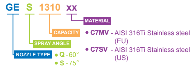
Flat fan nozzle - EU GES 1310 C7MV
